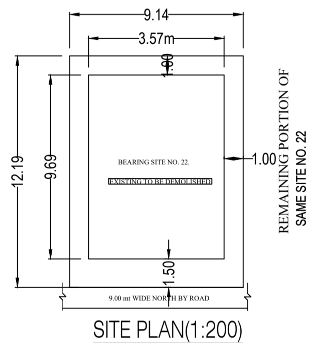
SITE PLAN (1:200)
